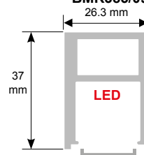
Cache BMS365/80 (droit uniquement right only - nur rechts)
